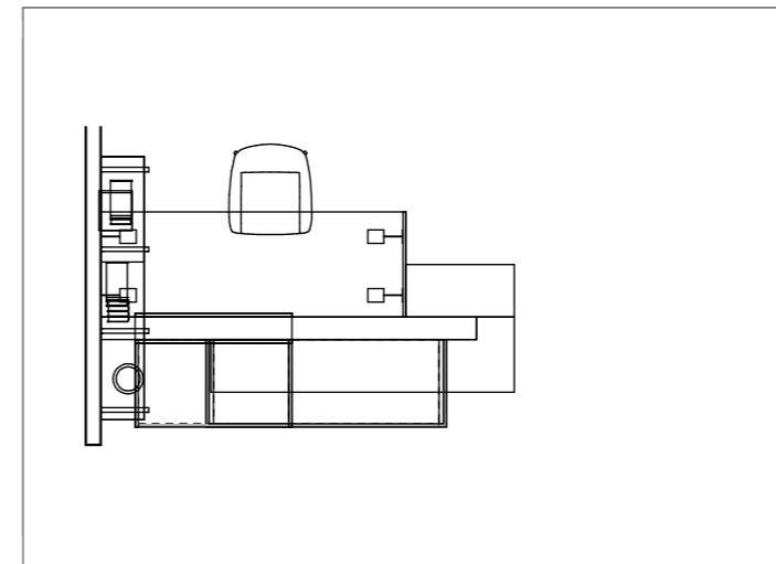
Kojen-Maße | Dimensions | Box | Kooi 2150 mm x 2750 mm
