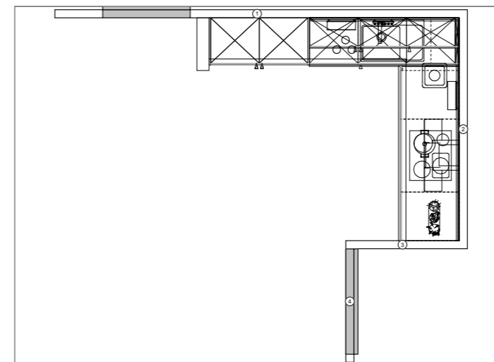
Kojen-Maße | Dimensions | Box | Kooi 3350 mm x 2750 mm
